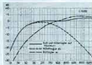
Frequenzgang bei verschiedenen Baß- und Höhenreglerstellungen
