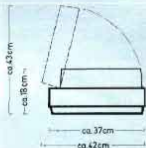
Skizze Studio 1520/Studio 1600
